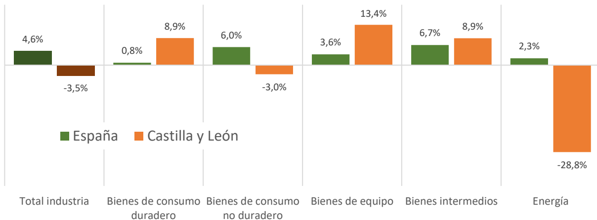
Gráfico 15. Variación anual de la producción industrial por destino económico de los bienes. Diciembre de 2024
